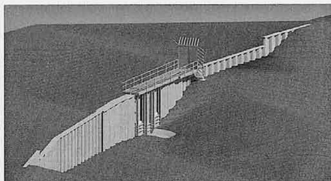
▲ 3D-Darstellung Siel
