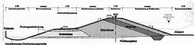
▲ Deichquerschnitt
