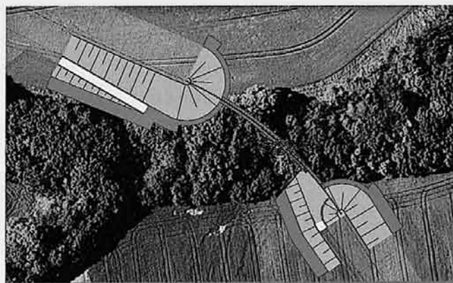
▲ Detaildarstellung Lageplan Siel Gelbes Wasser auf Luftbild
